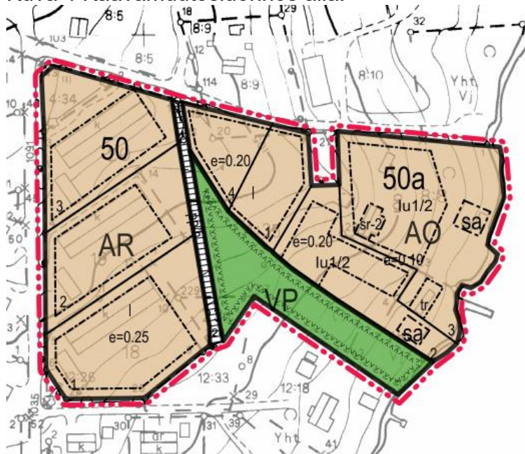
Kuva 4 Kaavamuuosluonnos alla:
